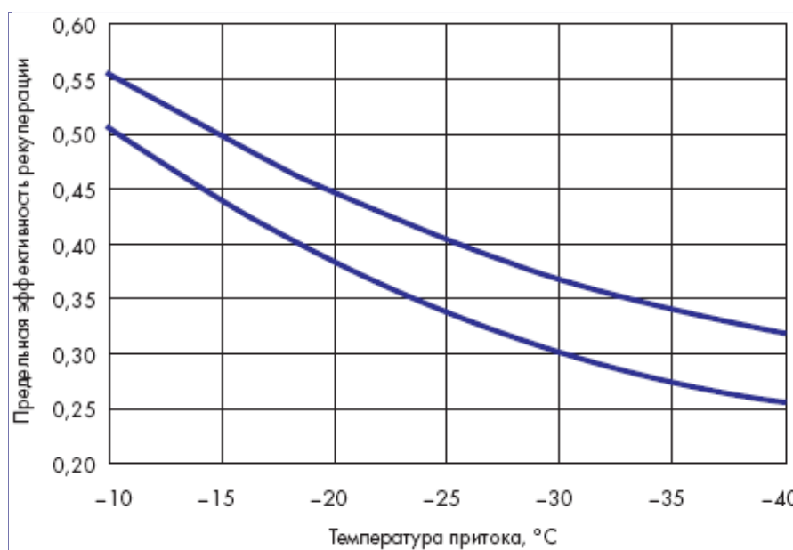
Рисунок 2. Предельная эффективность по условиям обмерзания
