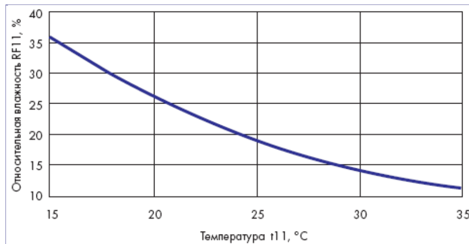
Рисунок 1. Нижний предел влажности по опасности обмерзания
